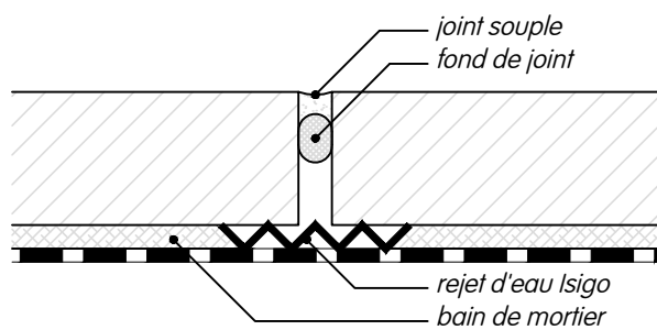
Joint couvre mur avec profil-isigo (par des tiers).
