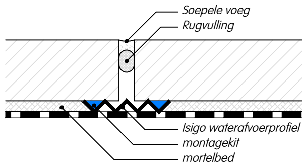
Sluiting voeg deksteen met isigo-profiel (door derden).
