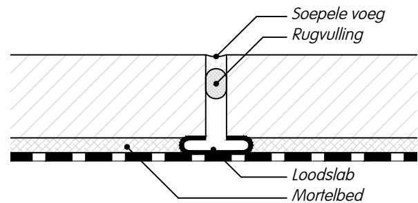
Sluiting voeg deksteen met loodslab (door derden).
